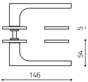
M269RB8B M269RY8B
